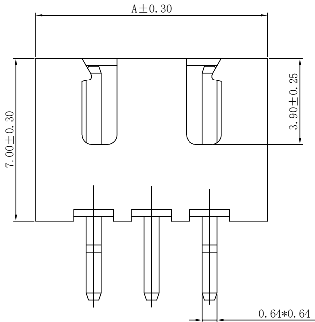
3P视图
