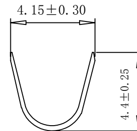
SEC A--A
