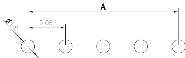
PCB安装尺寸图
