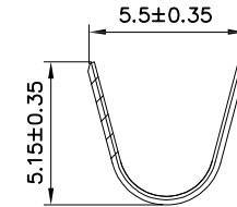
高脚12AWG
